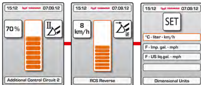
Einstellung der Ölmenge des dritten und vierten Kreises über das Display.
